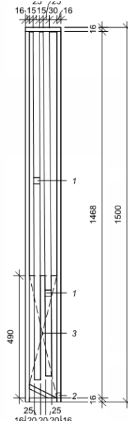
2 Doorsnede
