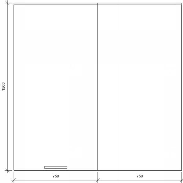
3 Vooraanzicht
